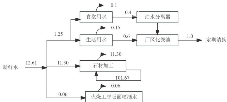
图2-3 扩建后全厂水平衡图 单位：m³/d
