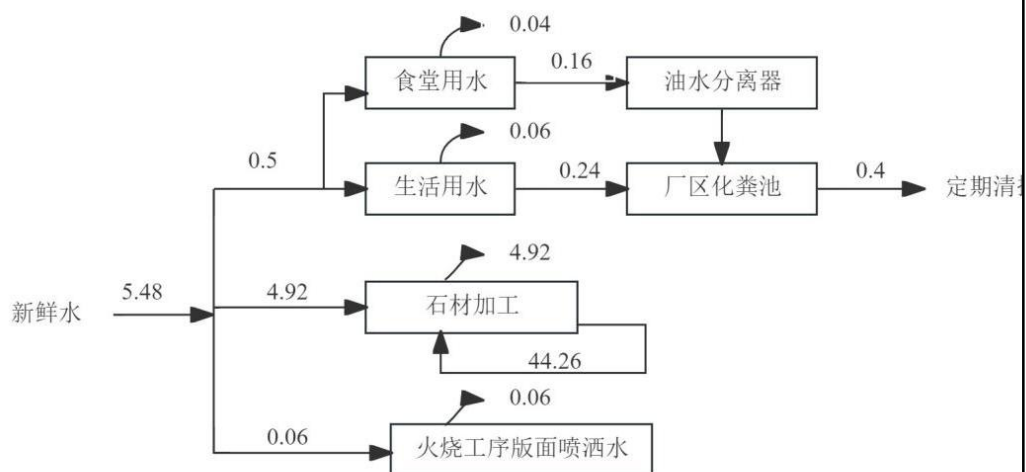
图2-2 扩建项目水平衡图 单位：m³/d
